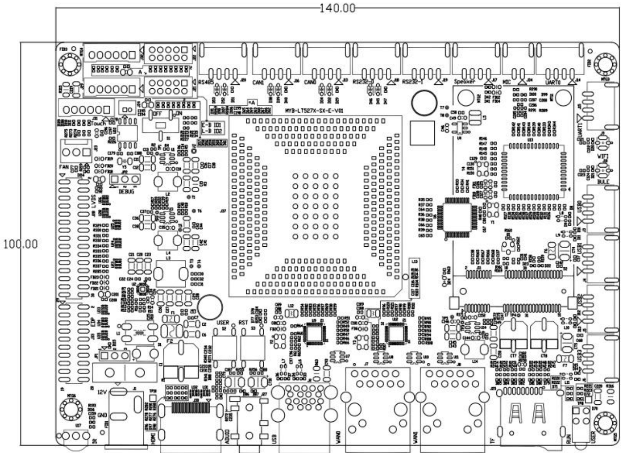
图 6-4 MYB-LT527M-SX 高清控制板机械尺寸图 (单位: mm)
