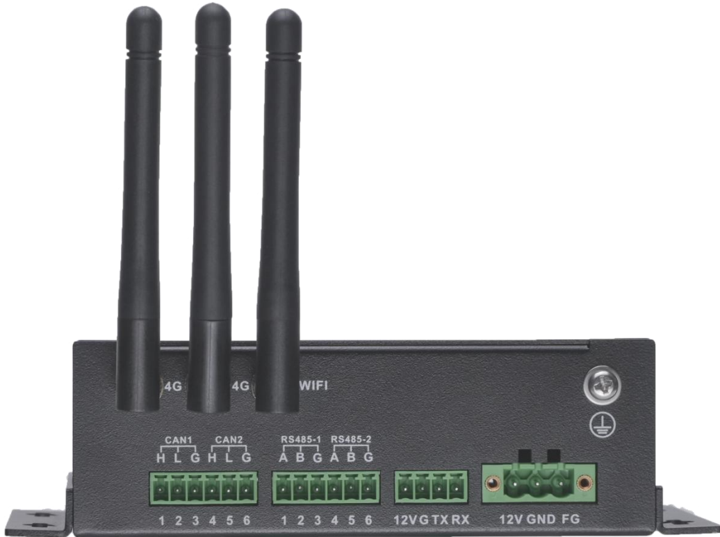
图 5-1 MYD-LT527M 开发板接口正面图
