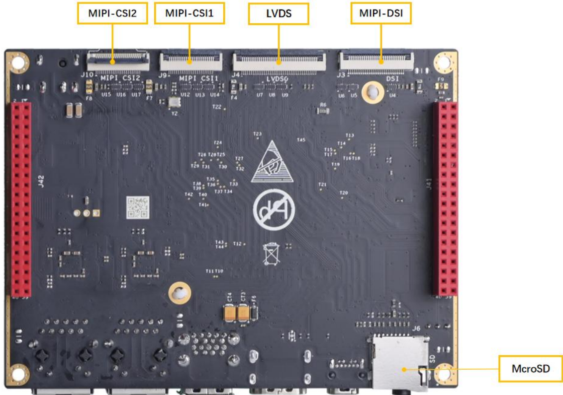
图 4-2 MYD-LT527M 开发板接口背面图
