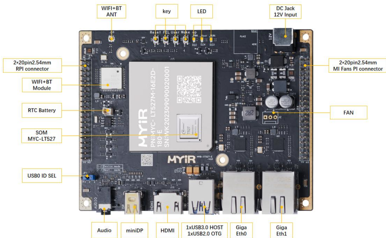
图 4-1 MYD-LT527M 开发板接口正面图
