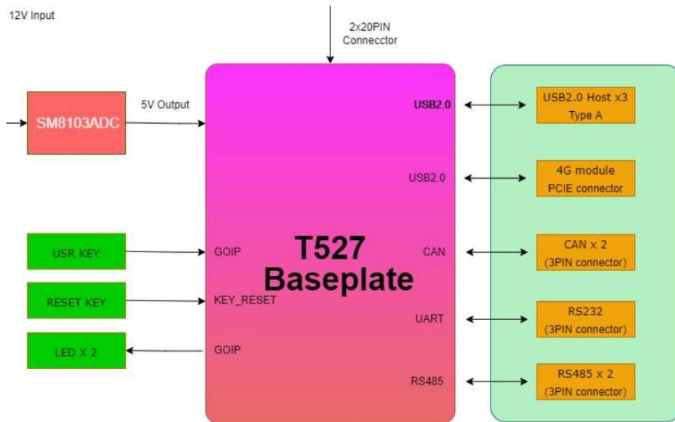
图 5-3 MYB-LT527M-I-GK-B 扩展底板系统框架图
