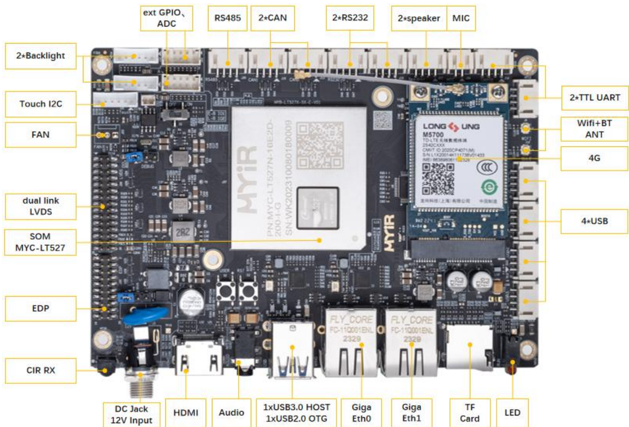
图 6-1 MYD-LT527M-SX 高清控制板接口正面图
