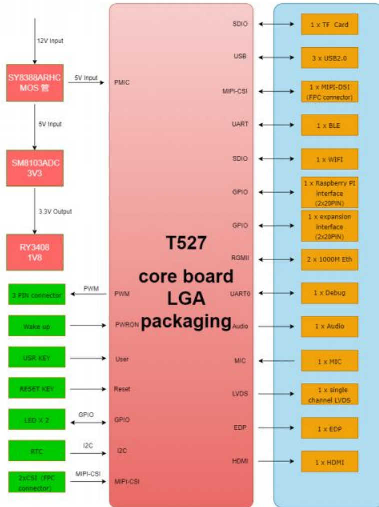
图 4-3 MYD-LT527M 开发板系统框架图
