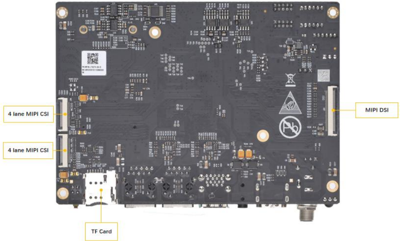
图 6-2 MYD-LT527M-SX 高清控制板接口背面图
