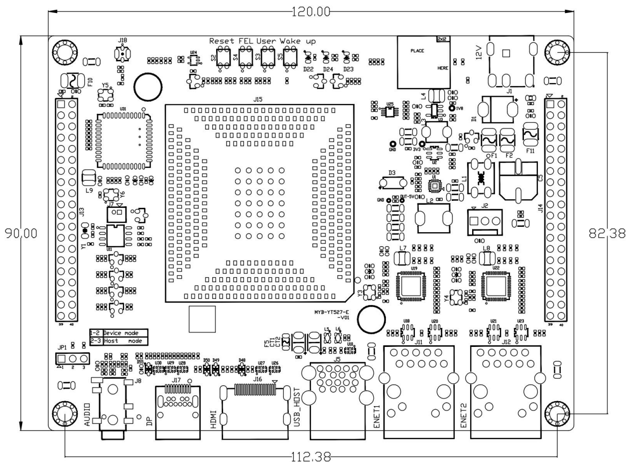
图 4-4 MYB-LT527M 机械尺寸图 (单位: mm)
