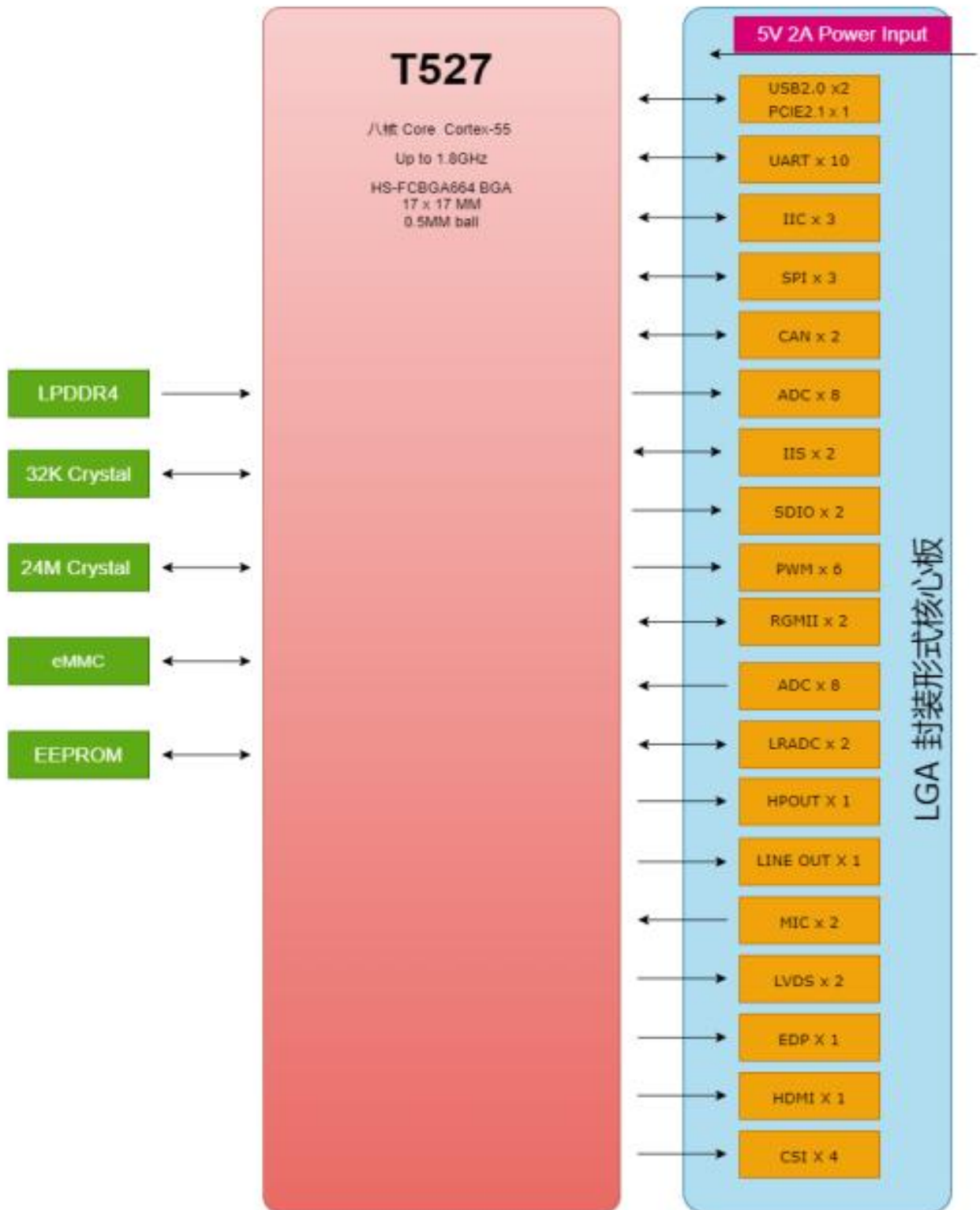
图 3-5 MYC-LT527M 核心板系统框图
