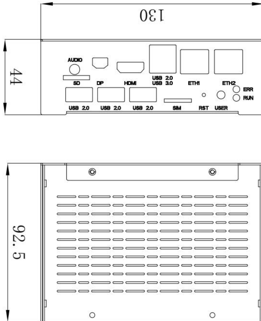
图 5-4 MYB-LT527M-I-GK-B 微型工控机机械尺寸图 (单位: mm)
