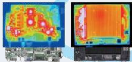
利用热成摄像头拍摄进行热分布分析
